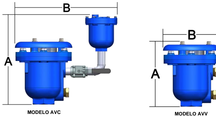
Figura 4. Dimensiones de válvulas AVV y AVC
