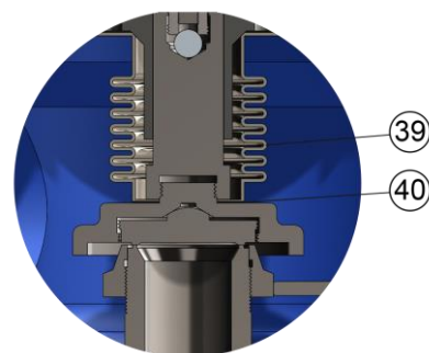
CONSTRUCCIÓN BALANCEADA
