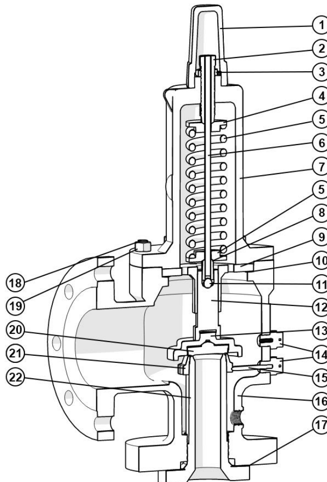
Fig.1 Seccionado de válvula de seguridad modelo 34A estándar.
